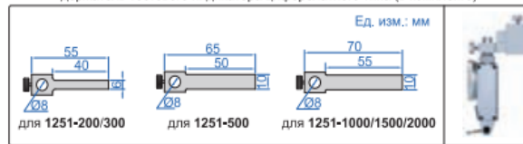
держатель тестового индикатора циферблатного типа (в комплекте)
