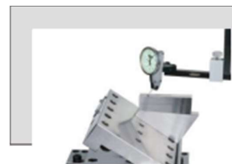
Установка угла пластины
